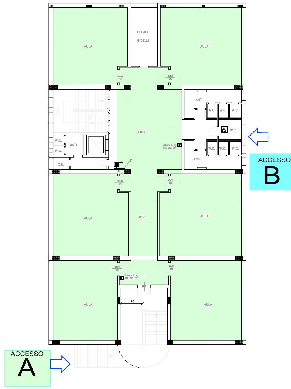
PIANO PRIMO
